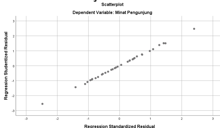
Gambar 1.1 Uji Heteroskedastisitas
