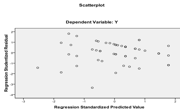
Gambar 2. Grafik Scatterplot
